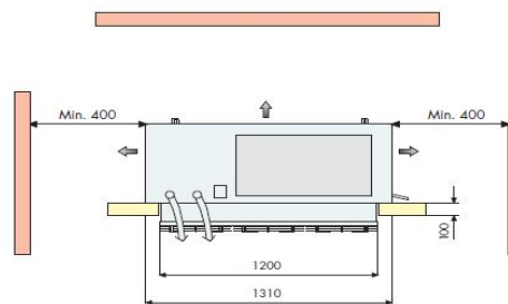
Disegno b Drawing b
