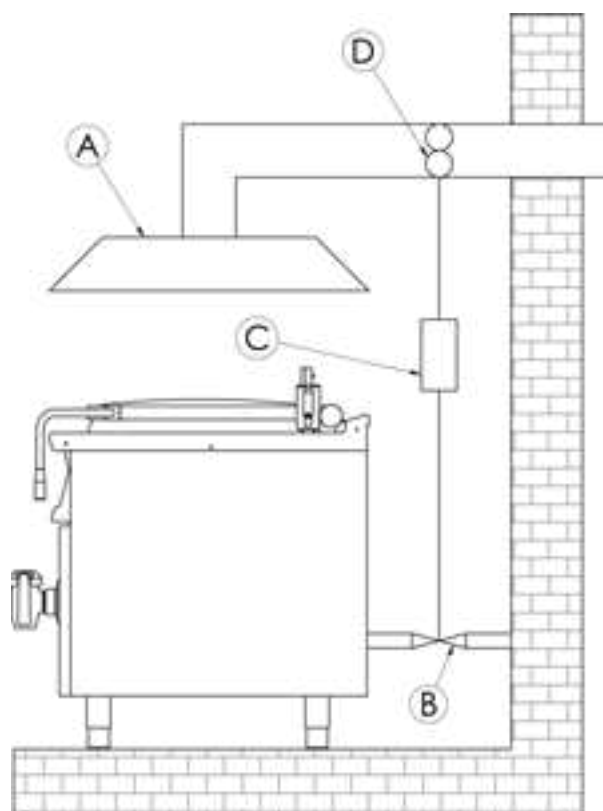
ABSAUGANLAGE
